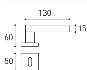
Maniglia con rosetta e bocchetta quadrata Door handle with square rosette and key hole
