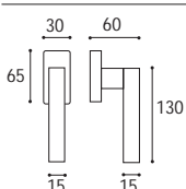
Maniglia per finestra DK \text{K} 7 \times 40 rosetta rettangolare Window handle DK \text{K} 7 \times 40 rectangular rose
