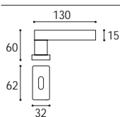
Maniglia con rosetta e bocchetta rettangolare Door handle with rectangular rosette and key hole
