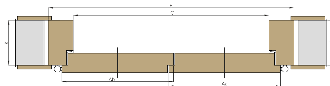
Double vantail avec feuillure avec huisserie fixe
