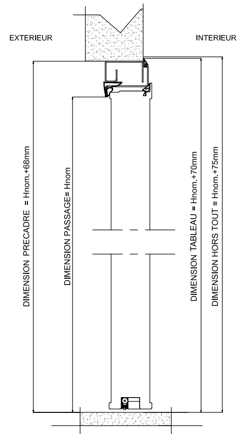
COUPE VERTICALE
