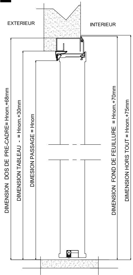
COUPE VERTICALE
