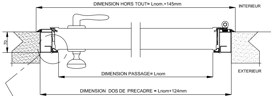
COUPE HORIZONTALE
