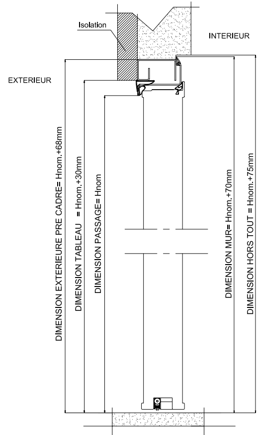
COUPE VERTICALE
