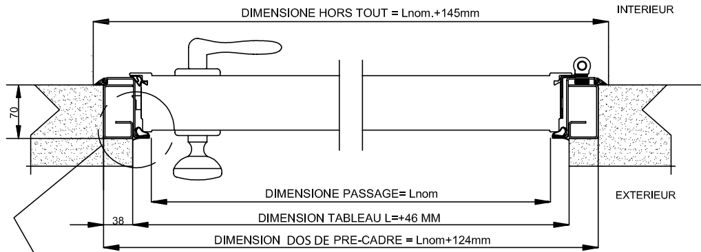
COUPE HORIZONTALE
