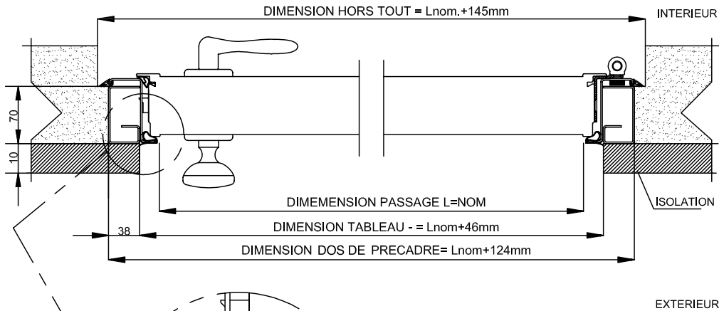
COUPE HORIZONTALE
